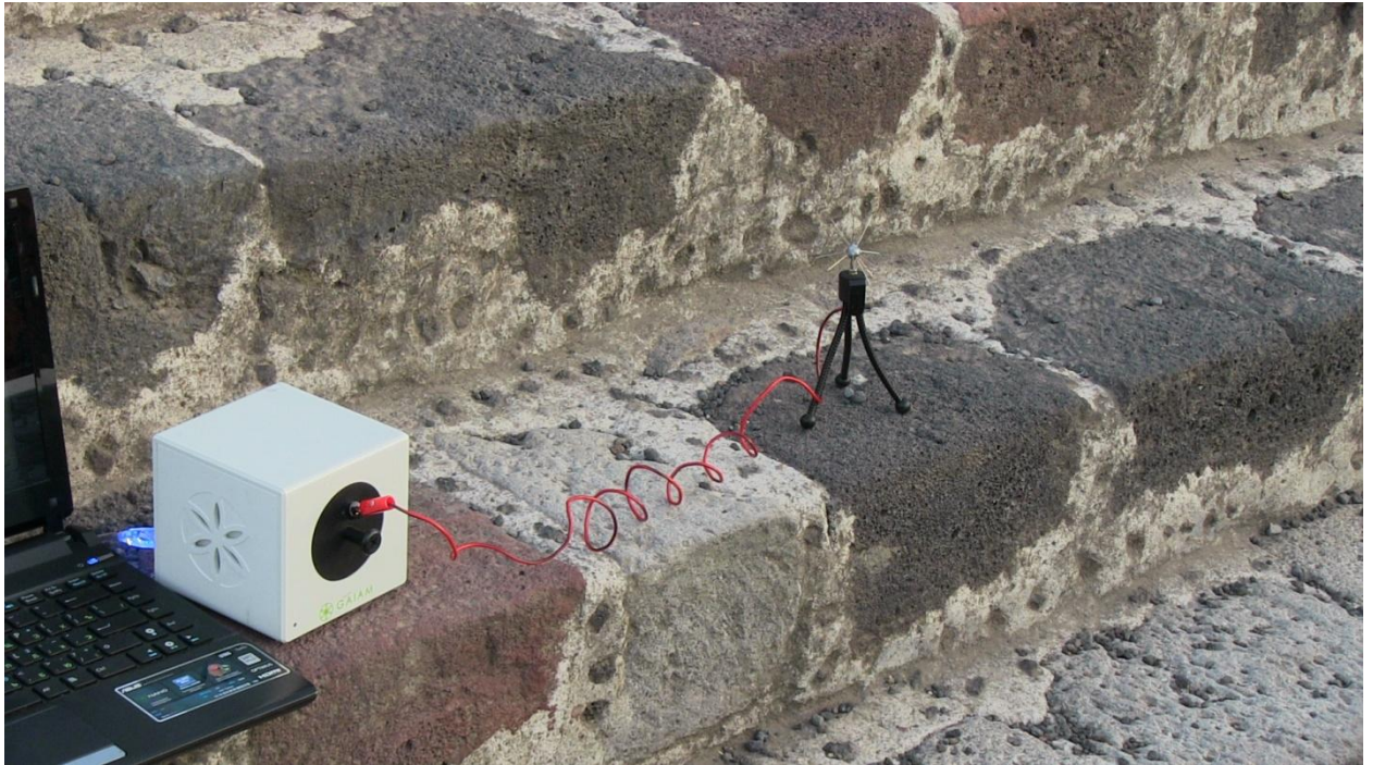
Fig.1. Sputnik sensor.
